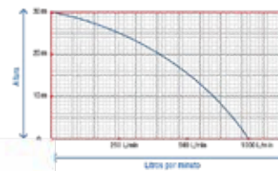
CURVA DE CAUDAL
